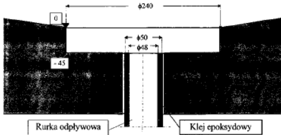
Rys. 9 Szkic sposobu osadzenia sączka - Wariant III - Etap II
