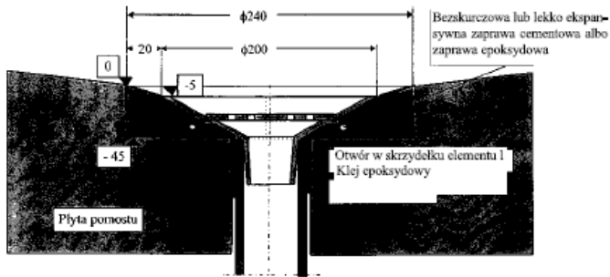
Rys. 10 Szkic sposobu osadzenia sączka - Wariant III - Etap III
